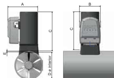
Propulsor Elétrico de Túnel CT100
